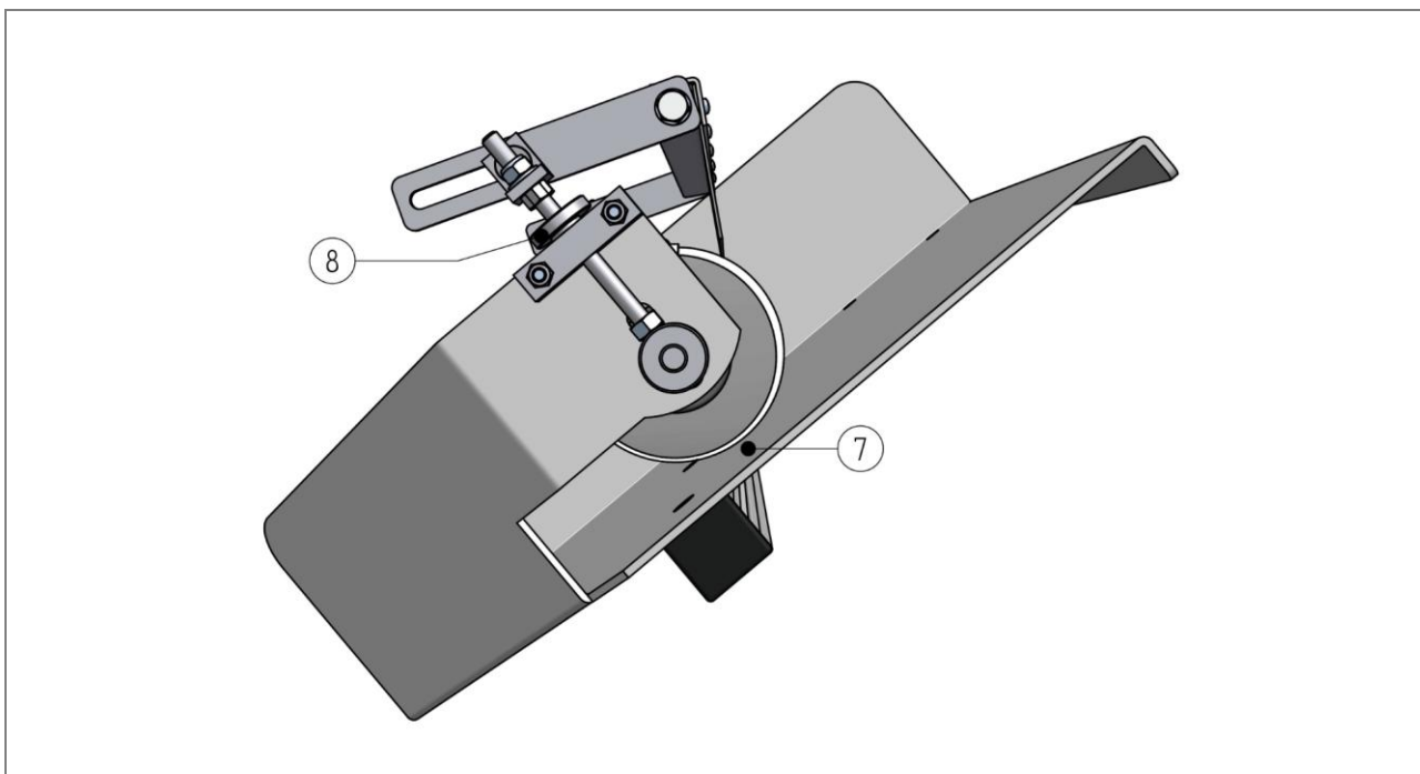
Fig. 6 : Vue latérale avec fente de séparation
