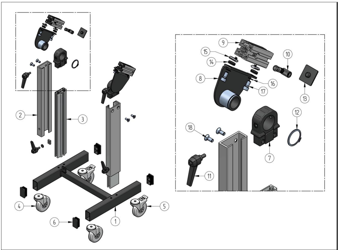
Fig. 16 : Bâti MSL/MSR
