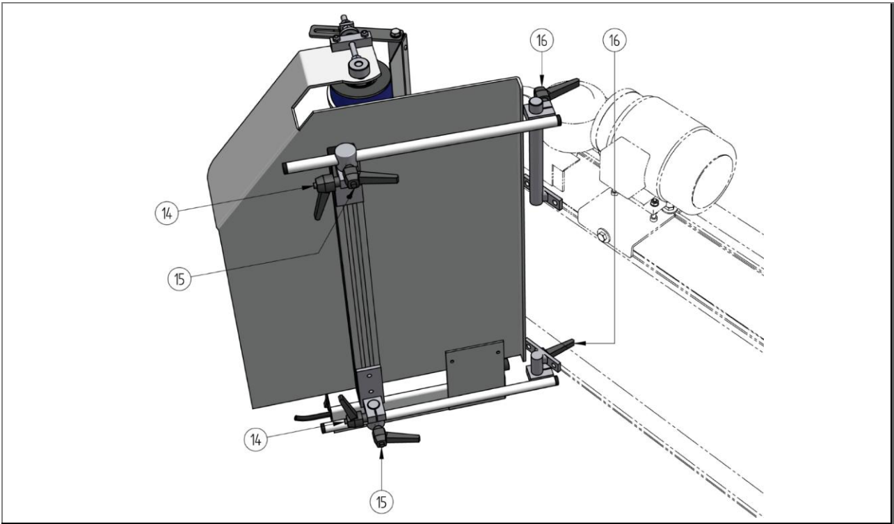
Fig. 10 : Cadre SAL/SAR
