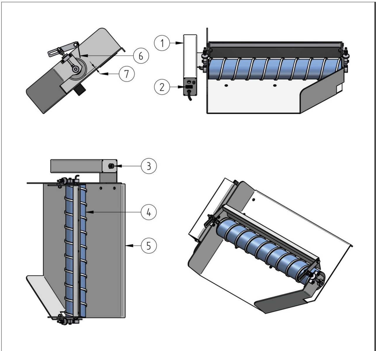
3. ábra: A csigás szeparátor teljes áttekintése
